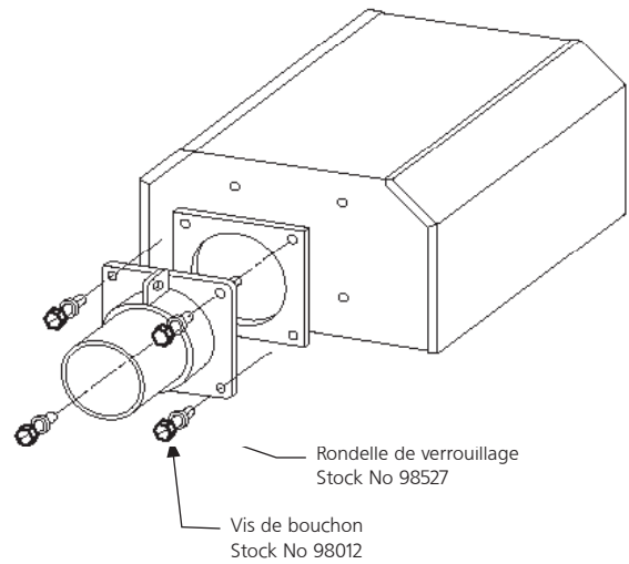
FIGURE 8 : Détail de la boîte du brûleur/Tube de transition
