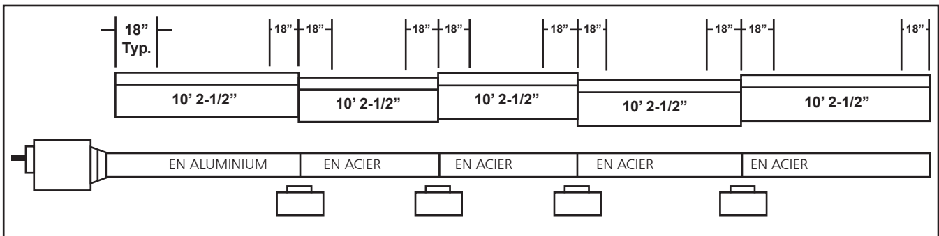
FIGURE 2G : Modèle Heatstar AG Heatstar AG Model HSAG-150, HSAG-175
