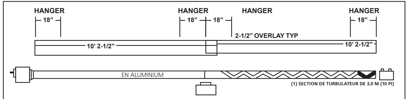
FIGURE 2C : Modèle Heatstar AG Heatstar AG Model HSAG-80
