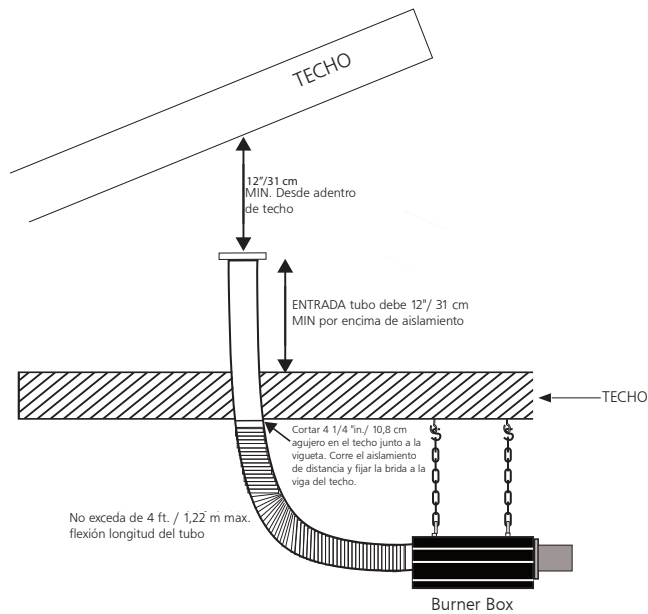
Figura 11: Entrada de aire desde el attillo
