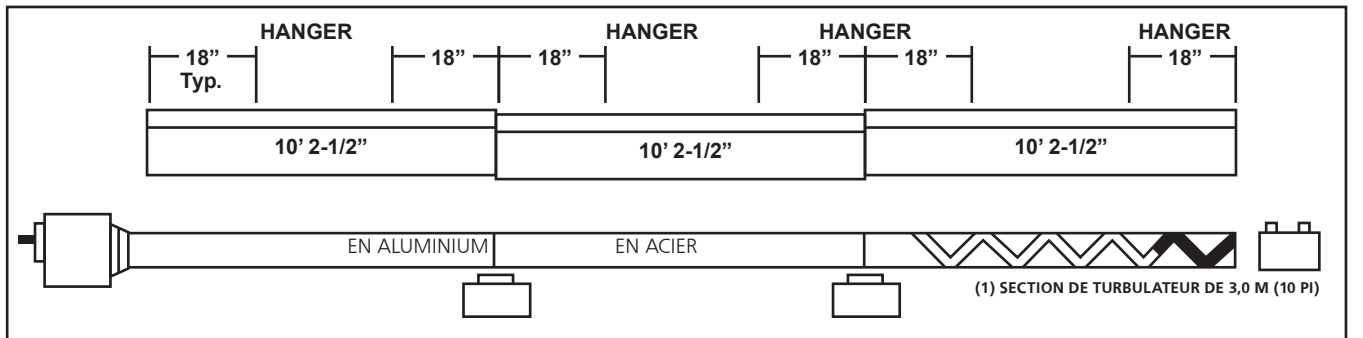
FIGURE 2D : Modèle Heatstar AG Heatstar AG Model HSAG-100
