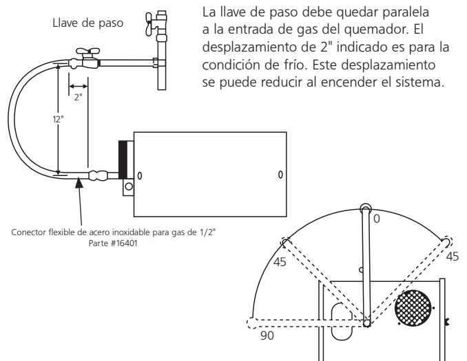
FIGURA 13: Conexión de línea de gas con conector de acero flexible para gas
