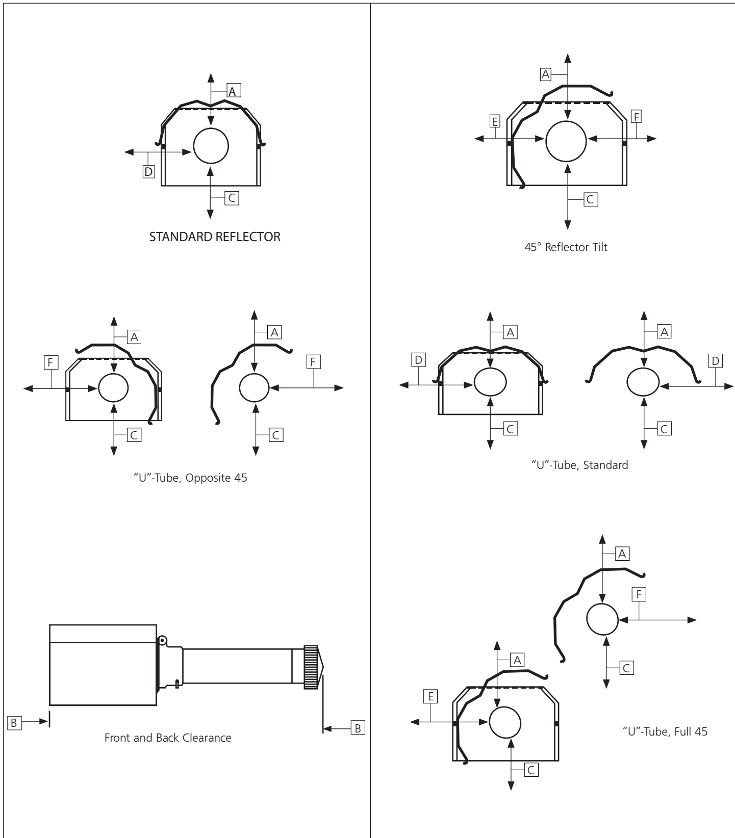
Figure 1 : Espaces libres aux combustibles (voir le TABLEAU 1 à la page 4)
