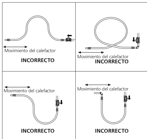
FIGURA 12: Conexión incorrecta de línea de gas con conector de acero flexible para gas
