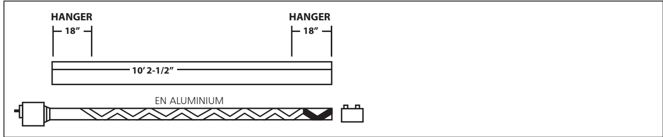
FIGURE 2B : Modèle Heatstar AG Heatstar AG Model HSAG-60, HSAG-80
